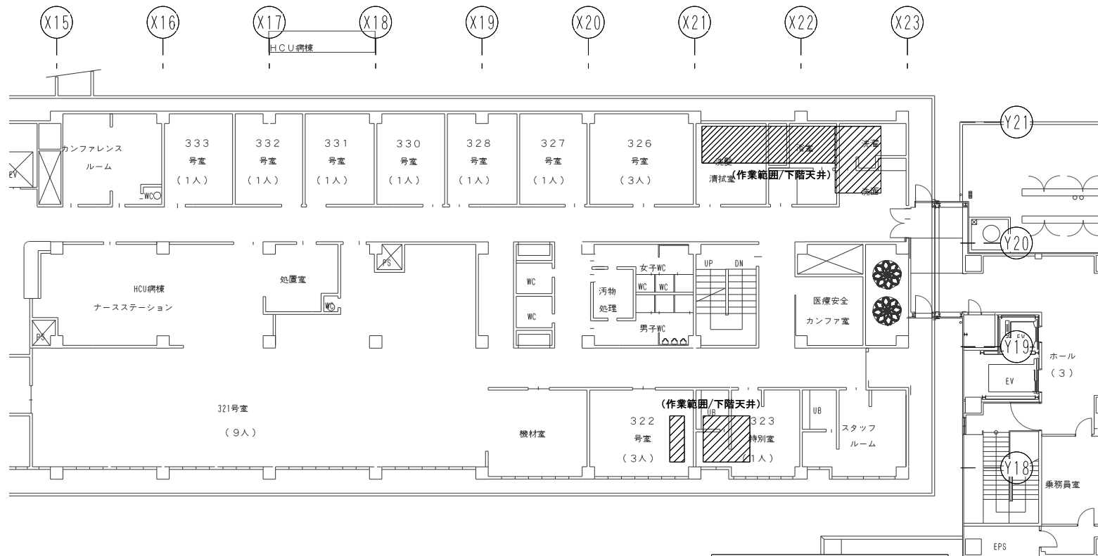
がんセンター棟 3階平面図
