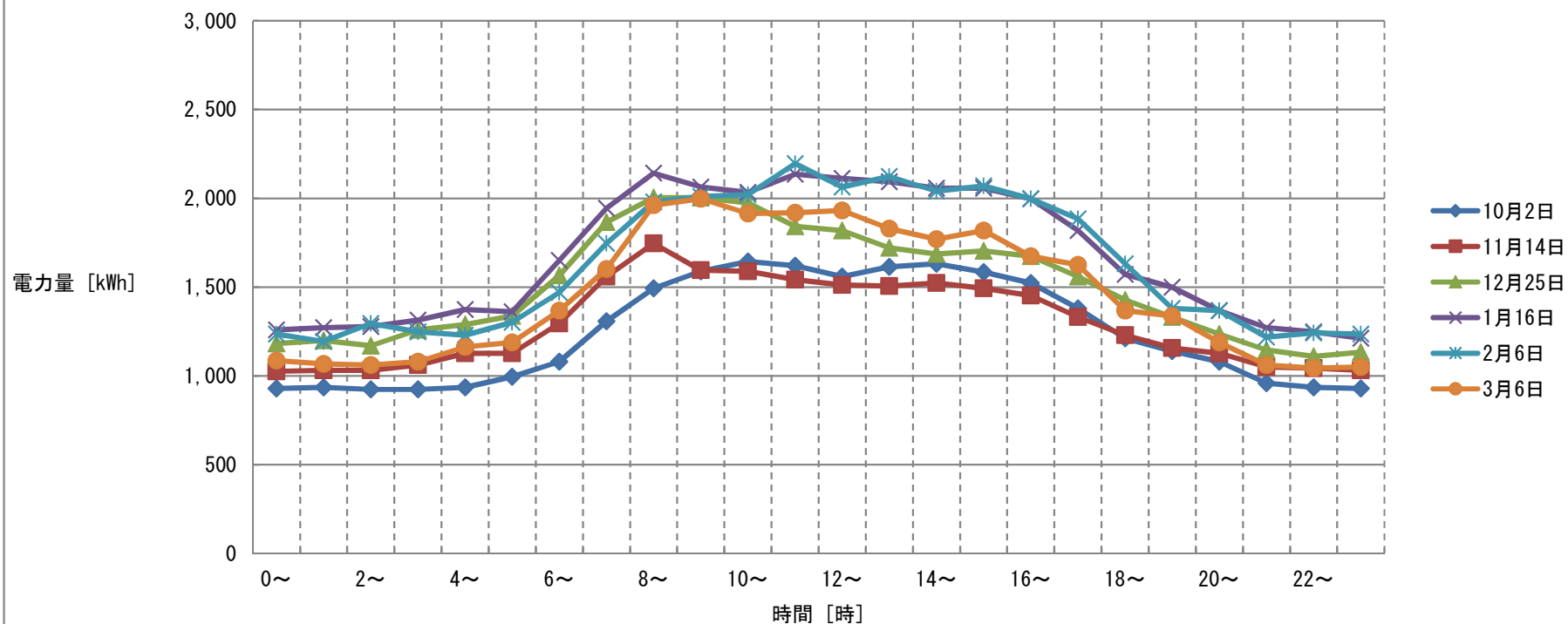
【茨城県立中央病院】月別最大負荷日ロードカーブ（令和5年10月～令和6年3月）
