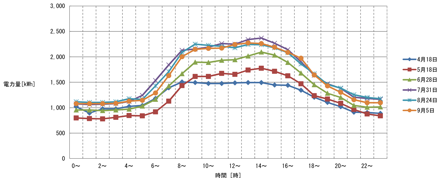
【茨城県立中央病院】月別最大負荷日ロードカーブ（令和5年4月～令和5年9月）
