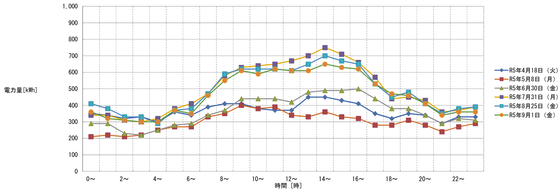
【茨城県立こころの医療センター】月別最大負荷日ロードカーブ（令和5年4月～令和5年9月）
