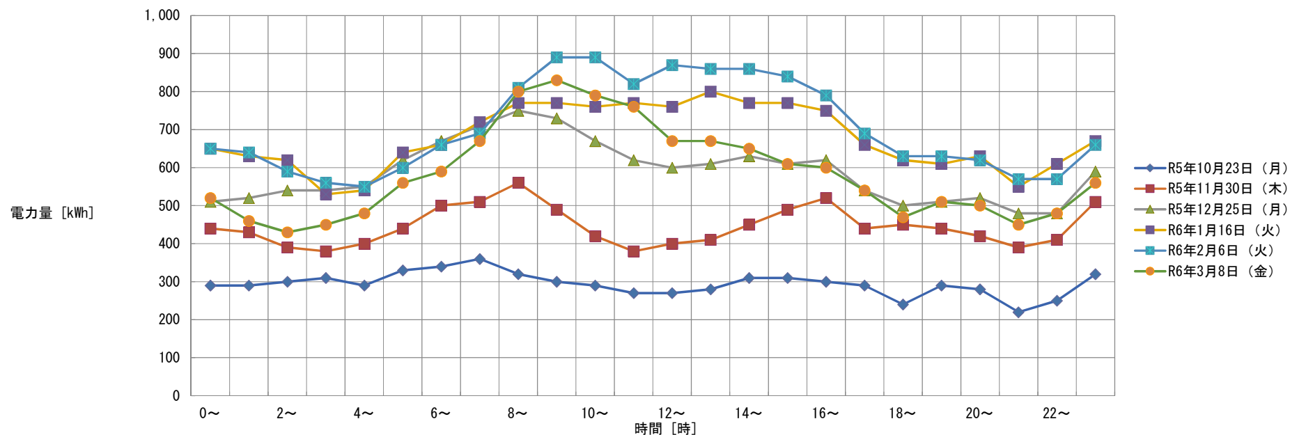
【茨城県立こころの医療センター】月別最大負荷日ロードカーブ（令和5年10月～令和6年3月）
