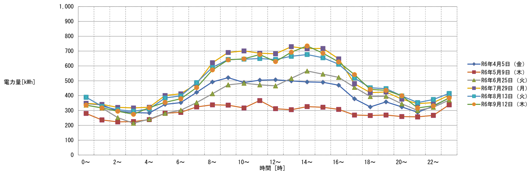
【茨城県立こころの医療センター】月別最大負荷日ロードカーブ（令和6年4月～令和6年9月）
