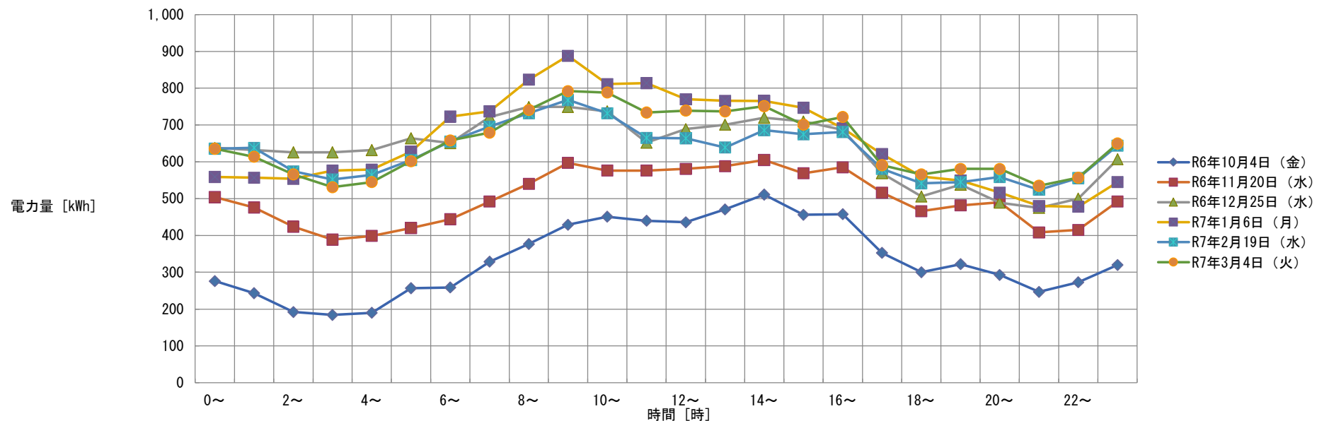
【茨城県立こころの医療センター】月別最大負荷日ロードカーブ（令和6年10月～令和7年3月）
