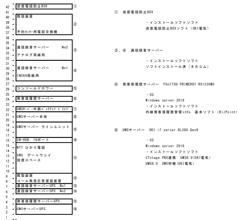
既設サーバーラック登録図 S: NS
